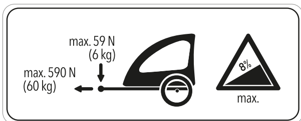
Afbeelding 44: Waarschuwingsticker aanhanger
