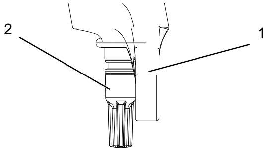
Afbeelding 71: Suntour trekdemperafsteller (2), vork (1)
