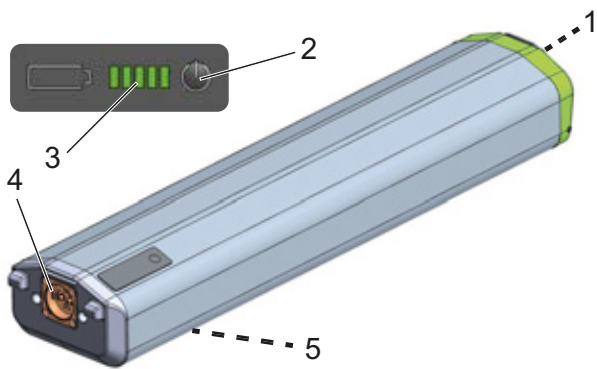
Afbeelding 13: Detail SuperCore accu
