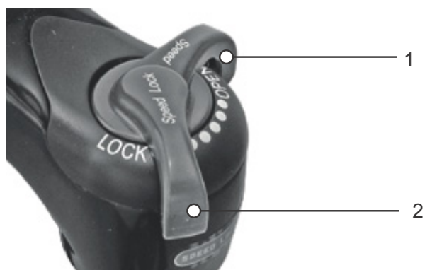
Afbeelding 62: Suntour drukdemper in open (1) en gesloten (2) stand
