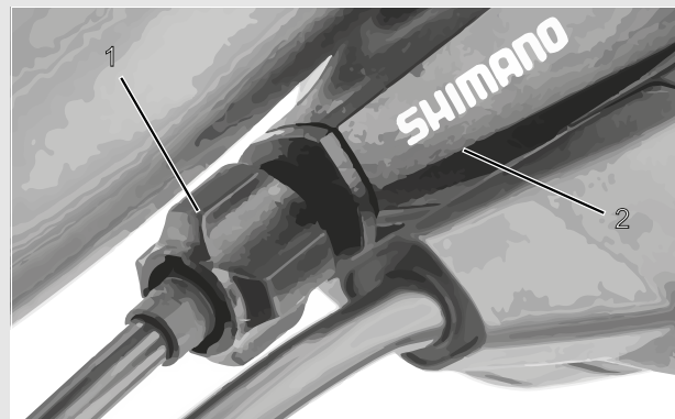
Afbeelding 67: Afstelwartel (1) van de versnelling met enkele bowdenkabelbediening en behuizing van de schakelhendel (2), voorbeeld
