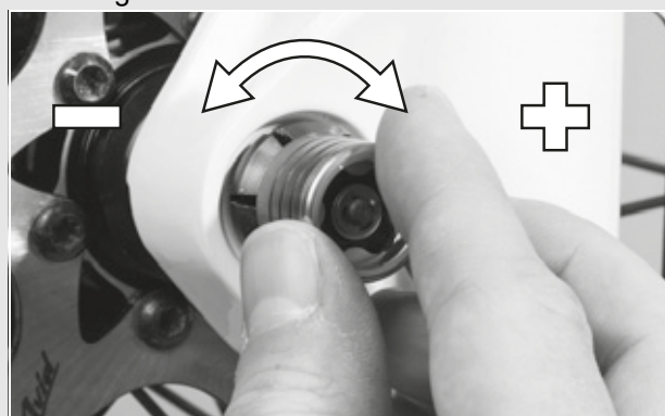
Afbeelding 31: Spanning afstellen
