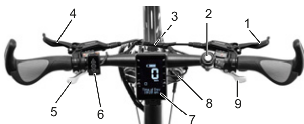
Afbeelding 16: Detailaanzicht pedelec vanuit berijderpositie gezien, voorbeeld
