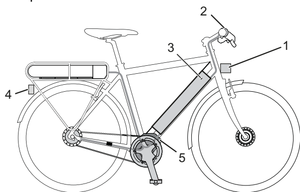
Afbeelding 12: Schema elektrisch aandrijfsysteem
