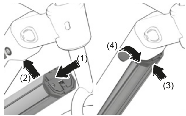
164 paveikslėlis. Integruoto akumulatoriaus įstatymas
