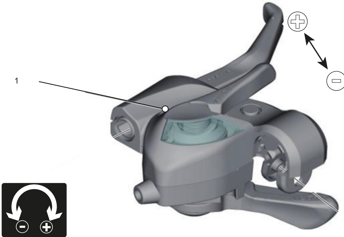
122 paveikslėlis. Nustatymo varžto guolis (1)
