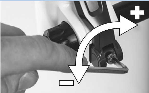
79 paveikslėlis. Ekscentriko įtempimo jėgos nustatymas
