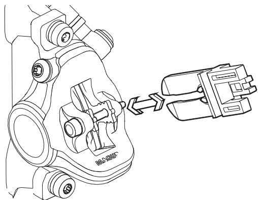
54 paveikslėlis. Transportavimo apsaugos tvirtinimas
