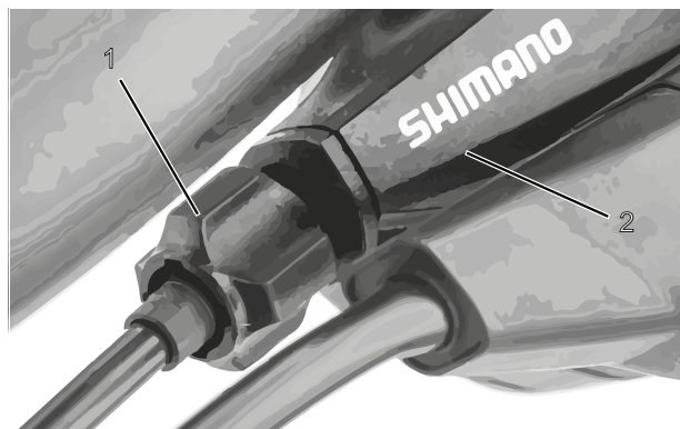
187 paveikslėlis. Reguliavimo įvorė (1) vieno praėjimo kabeliu valdomam pavarų perjungimui su pavarų svirties korpusu (2), pavyzdys
