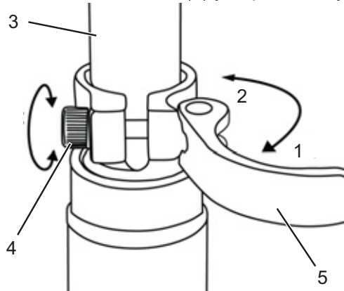
91 paveikslėlis. Balnelio atramos ekscentriko atidarymas
