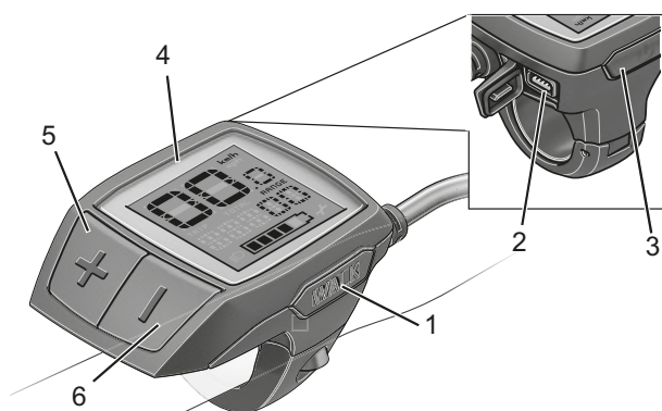
166 paveikslėlis. „BOSCH Purion“ borto kompiuterio konstrukcija
