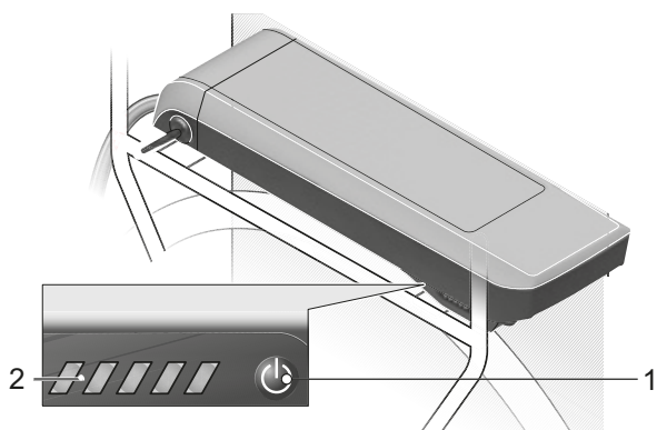
50 paveikslėlis. Bagažinės akumulatoriaus įkrovos būsenos indikatoriaus padėtis
