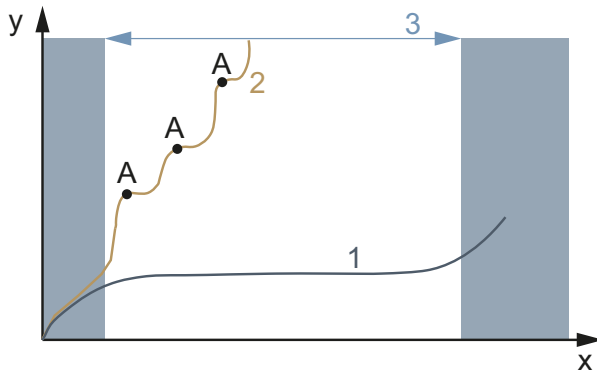
176 paveikslėlis. Diagrama: nusidėvėjimas, veikimo laikas (x) iki medžiagos pašalinimo (y)
