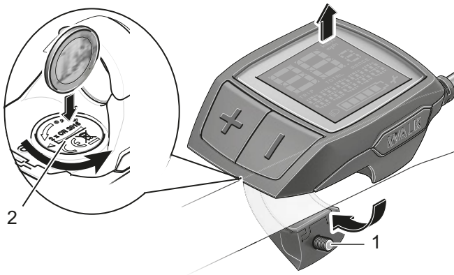
167 paveikslėlis. Borto kompiuteris su tvirtinimo varžtu (1) ir baterijų dėtuves dangteliu (2)
