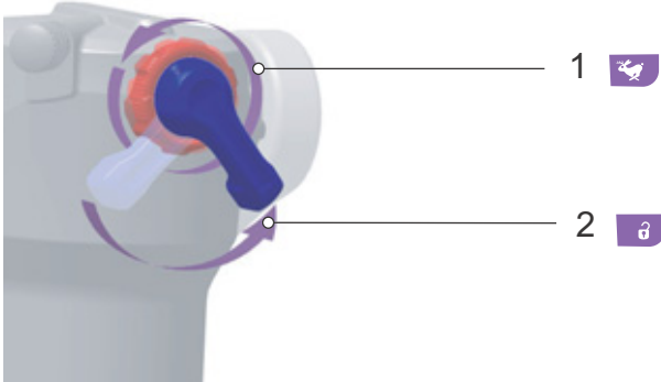
138 paveikslėlis. Atšokimo (1) ir kompresinio slopintuvo (2) atidarymas
