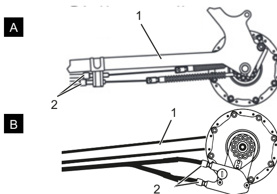
188 paveikslėlis. Dviejų pakopų, dviejų alternatyvių variantų (A ir B) reguliavimo įvovės (2), kabeliu valdoma pavarų perjungimo grandinės atrama (1)
