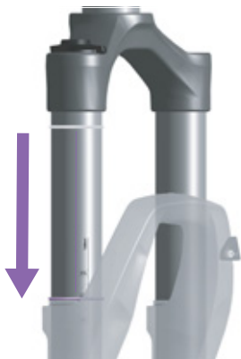
131 paveikslėlis. Žiedinės tarpinės pastūmimas ant amortizuojančių šakių
