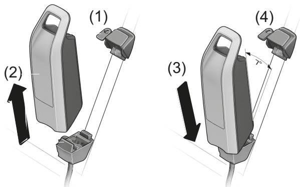
161 paveikslėlis. Rėmo akumulatoriaus ištraukimas ir įstatymas
