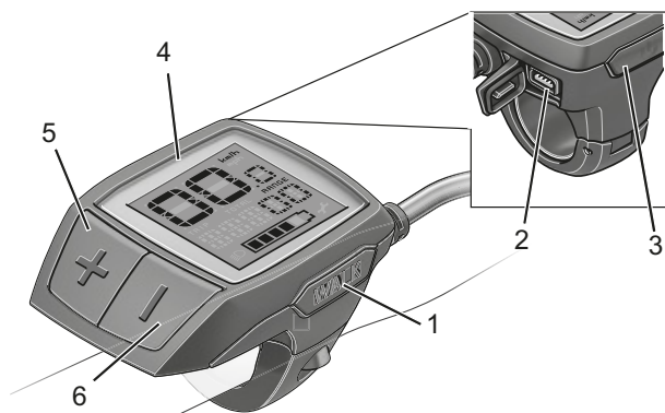
153 paveikslėlis. „BOSCH Purion“ borto kompiuterio konstrukcija
