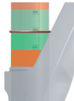
133 paveikslėlis. Normatyvinis SAG diapazonas (žalias) ir draudžiamas SAG diapazonas (raudona)
