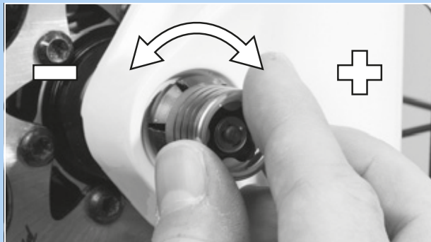
82 paveikslėlis. Įtempimo nustatymas
