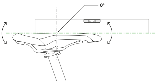
98 paveikslėlis. Horizontalus balnelio pokrypis su 0° pokrypiu balnelio viduryje
