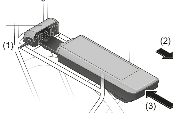
162 paveikslėlis. Bagažinės akumulatoriaus ištraukimas (2) ir įstatymas (3)
