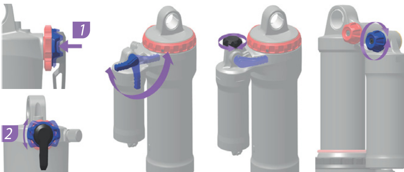
284 paveikslėlis. Kompresinio reguliatoriaus (mėlyna spalva) padėtis ir forma priklauso nuo modelio
